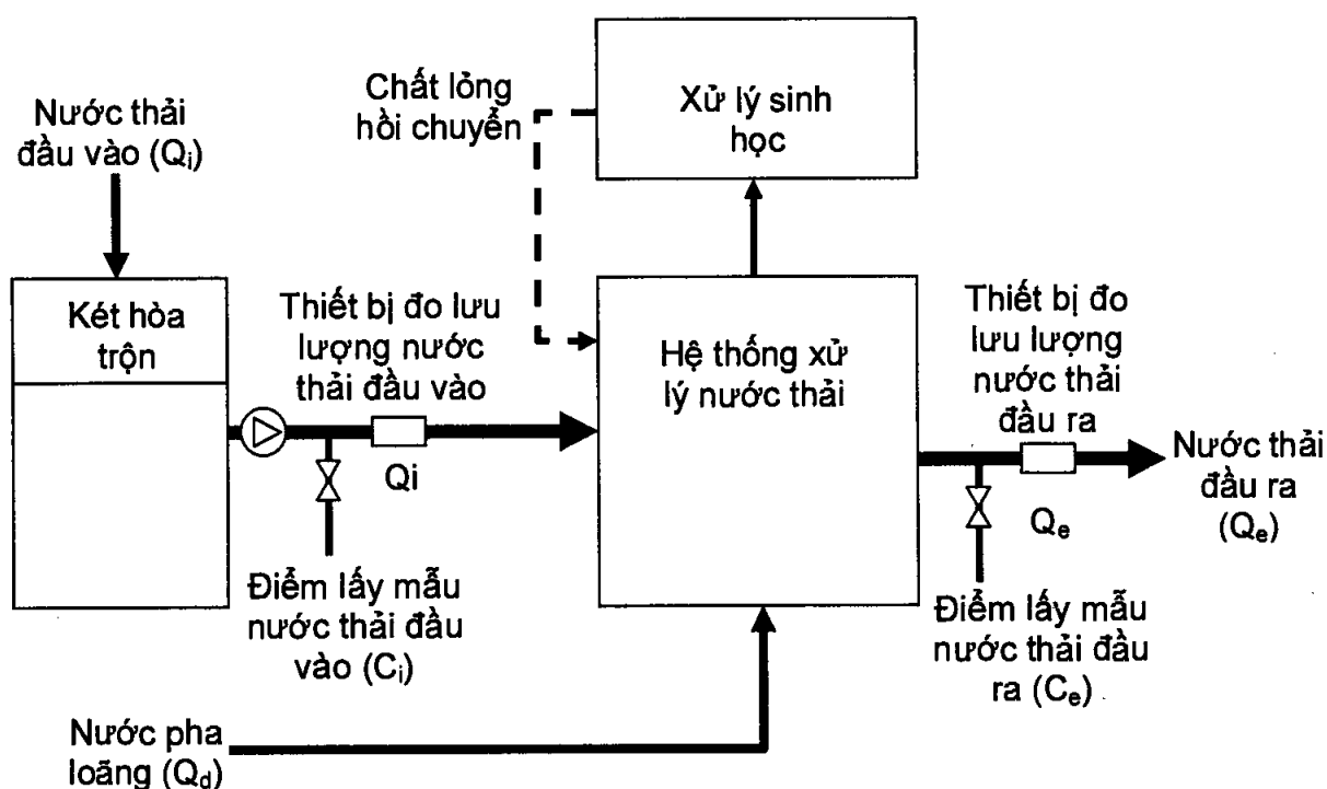
Hình 1. Sơ đồ hệ thống xử lý nước thải
