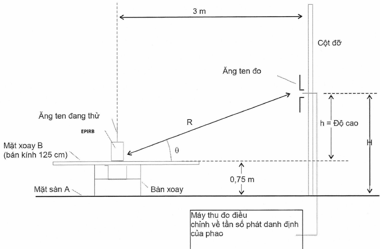
Hình 2 - Thiết lập đo kiểm
