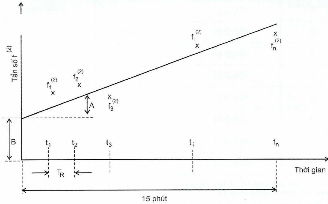
Hình 6 - Đo độ ổn định tần số thời hạn trung bình
